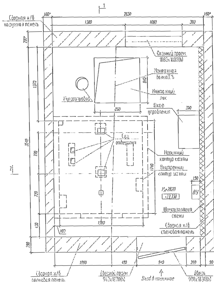
План машинного помещения
