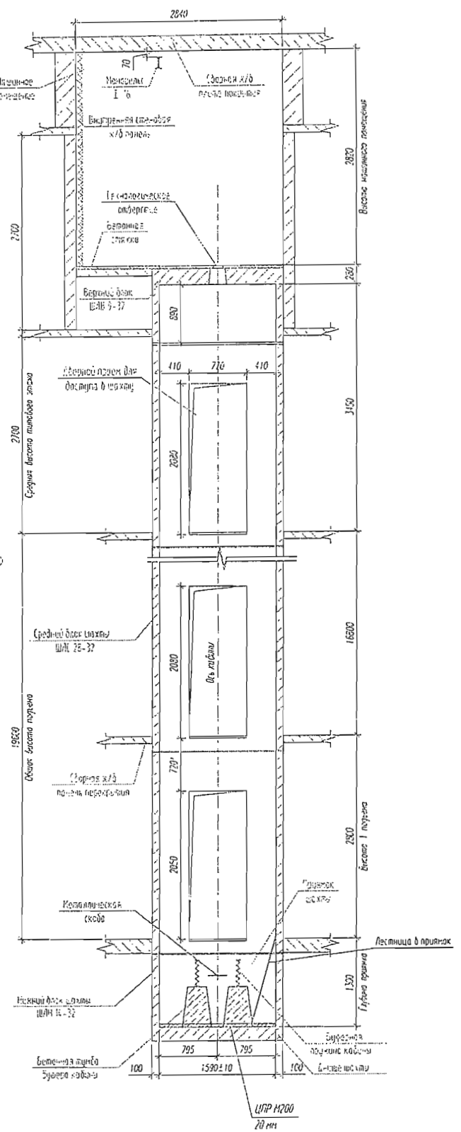
Разрез 2-2
