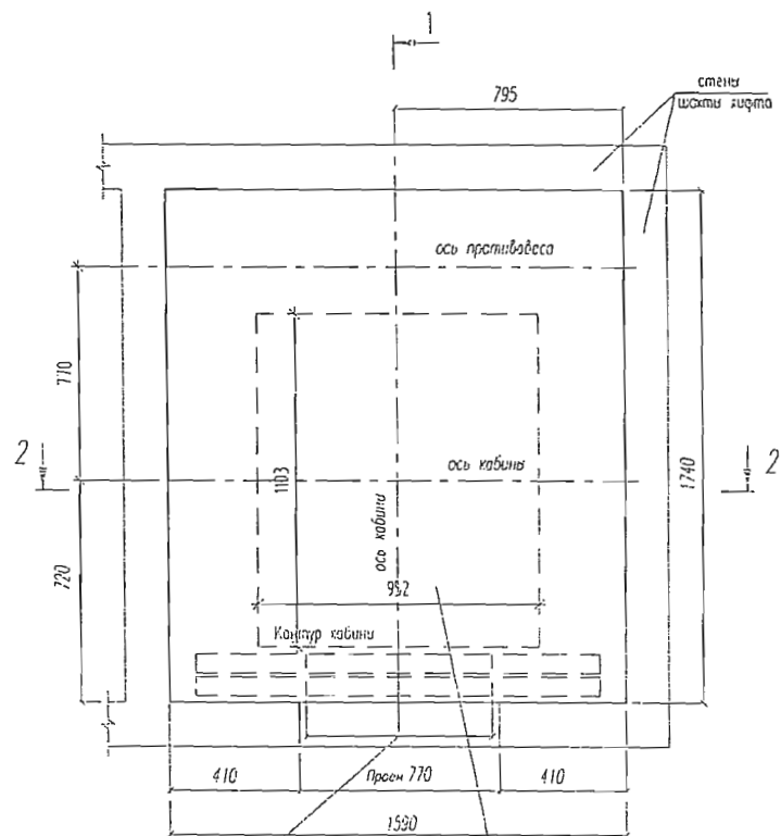
План шахты
