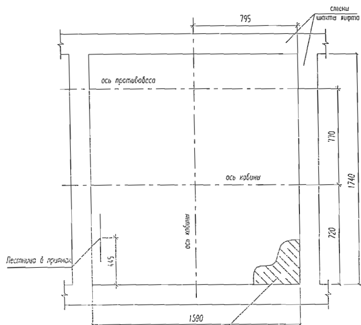
План приямка
